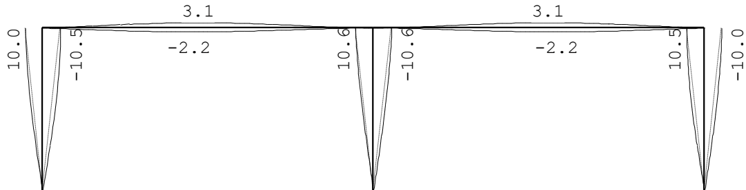
VERVORMINGEN W_{max} Frequente combinatie
