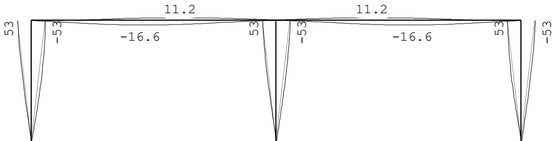
VERVORMINGEN W_{max} Karakteristieke combinatie
