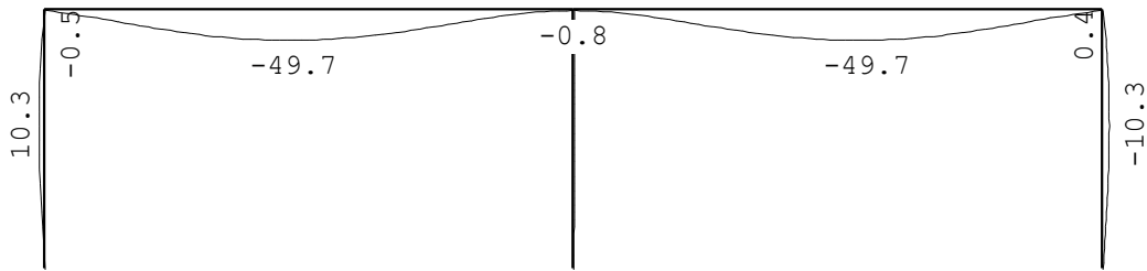
VERVORMINGEN W_{bij} Karakteristieke combinatie
