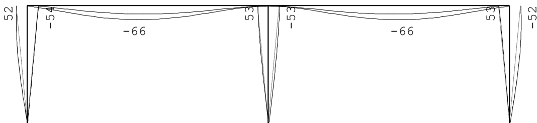
DOORBUIGINGEN Karakteristieke combinatie
